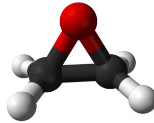
Etyleenioksidimolekyylin malli
