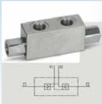
Kaksois paineen- rajoitusventtiili
