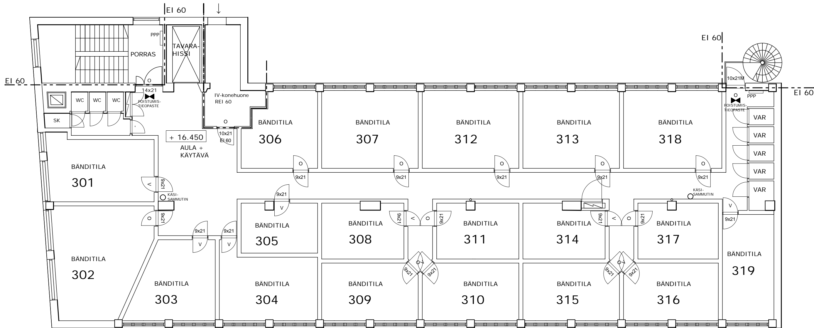
2. KERROS
