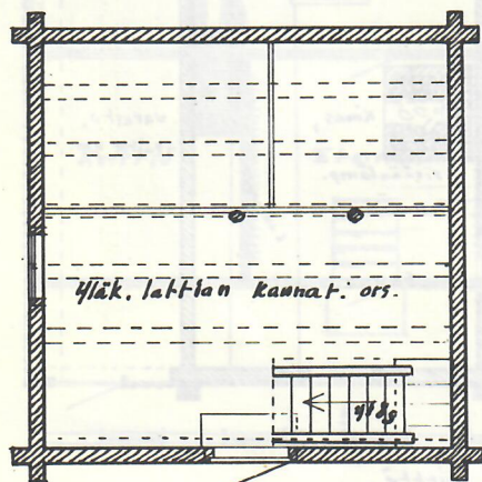
Aitta; pohjakaava.
