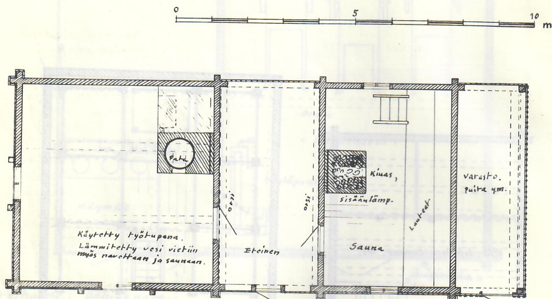
Saunarakennuksen pohjakaava. Osittain, hirttä, työtupa ja sauna, osittain lautarak, eteinen ja varasto. Työtupa ja saun vuorattu pystylautoituksella, ilman listoja. Takaseinä vuoraamaton. N. v. 1900.
