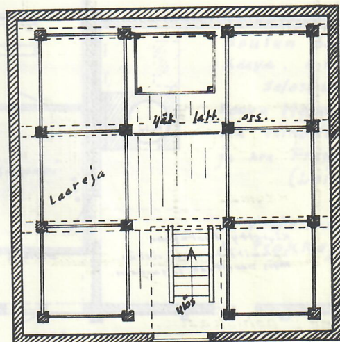
vilja-aitta; pohjakaava
