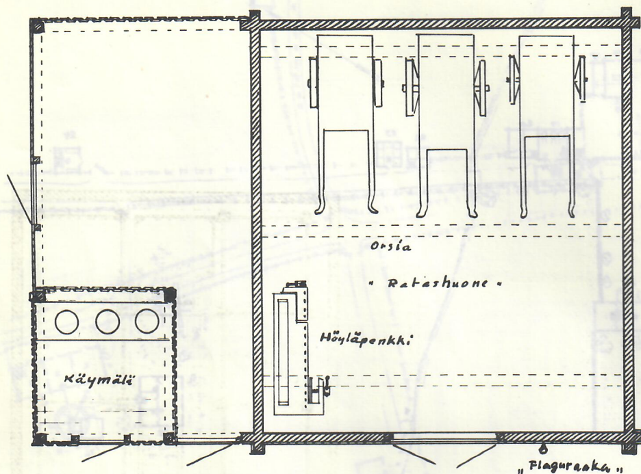
Ratashuone ; pohjakaava.
