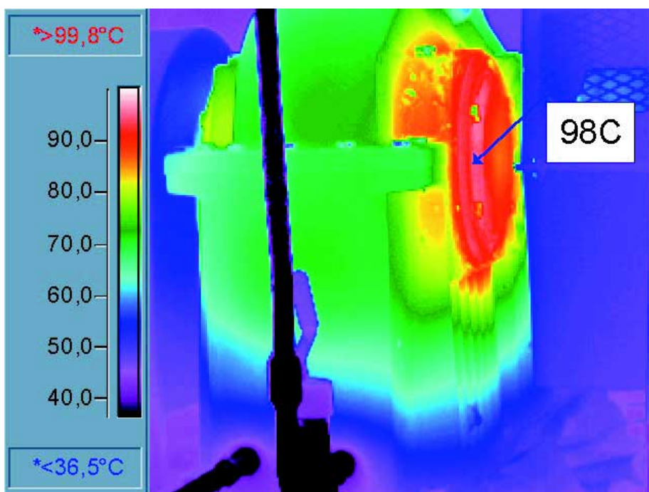
Kuva 1b. Viallinen laakeri.
