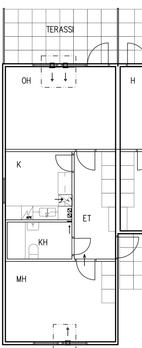
Huoneistotyyppi 2 1. kerros
