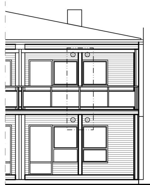
Julkisivuote huoneistotyyppi 2:n parvekkeiden ja terassien puolelta
