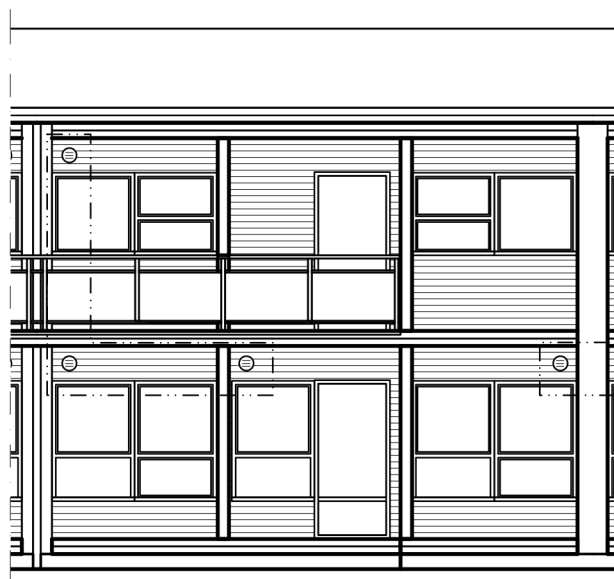
Julkisivuote huoneistotyyppi 5:n parvekkeiden ja terassien puolelta
