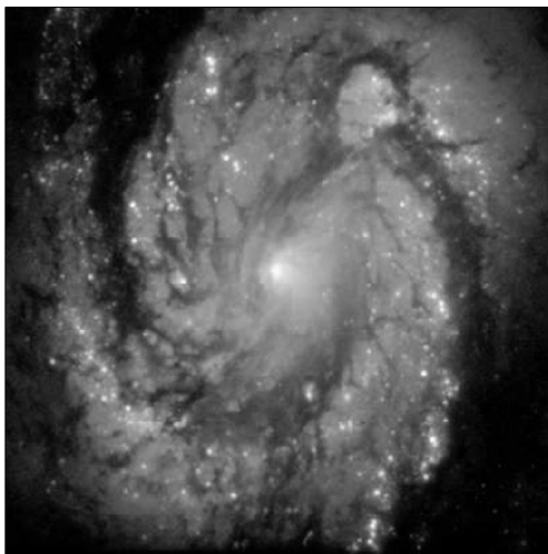
Tämä ajokoirien tähdistössä sijaitseva kierteisumu (galaksi) koostuu sadoista miljardoista tähdistä. Tämä on hyvin tyypillinen galaksi, jollainen myös oma linnunratamme on.
