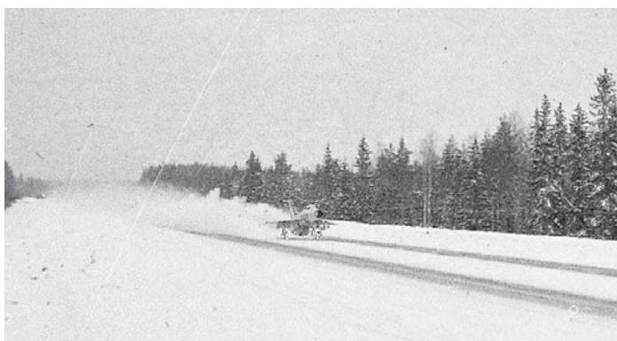
Lasku tehtiin tien keskiviivalle, joka oli lumikerroksen peitossa. Nokka mahdollisimman kauan ylhäällä ilmapirran hiljentäessä vauhtia. Jarruvarjoja ei käytetty, sillä tiellä riitti pituutta. Koneet rullasivat suoraan suojapaikkoihin, joissa tankkaukset. Kiitotiellä mahdollisimman vähän sotilastoimintaa, jotta ei olisi tultu paljastuneeksi tiedustelukoneille.
