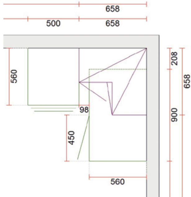
Piilokulma 900 mm
