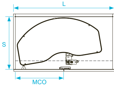
YLÄNÄKYMÄ
