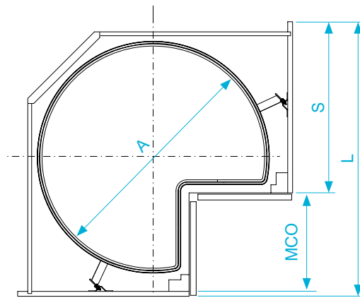
YLÄNÄKYMÄ
