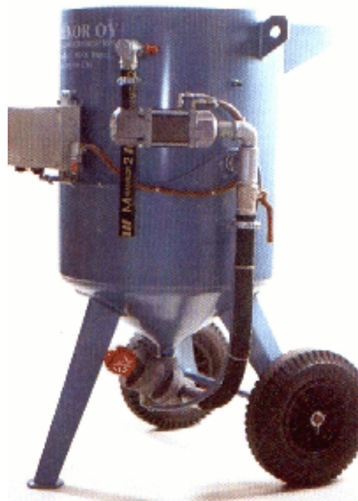
Paineastia 200 L, sähköinen kauko-ohjaus, Combo ohjausventtiili, Thompson paineilmaohjattu teräshiekkaventtiili
