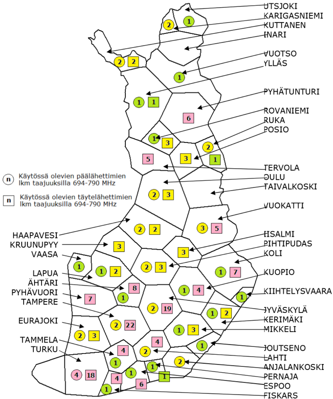
Kuva 14 Manner-Suomessa taajuusalueella 694-790 MHz käytössä olevien pää- ja täytlähettimien lukumäärä nimetyin päälähetin alueittain.
