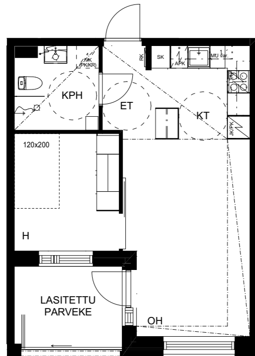
PERUSRATKAISU, 2H+KT
