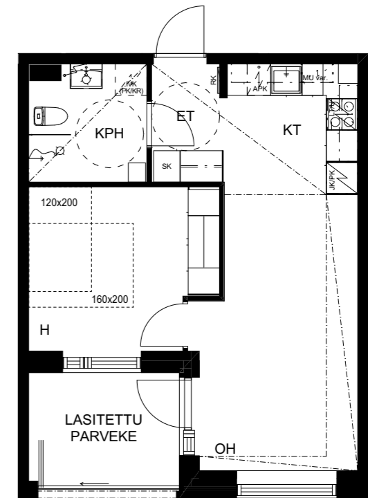
VAIHTOEHTO 3, 2H+KT
