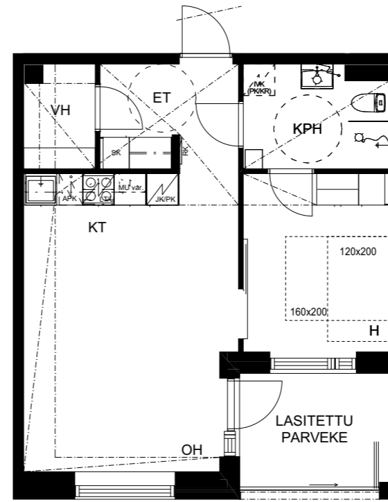
VAIHTOEHTO I, 2H+KT
