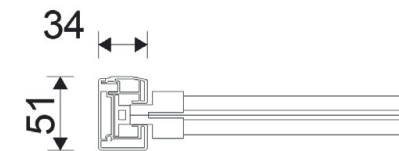
Sivukanaalin leikkaus päältä
