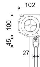
Asennus aukkoon
