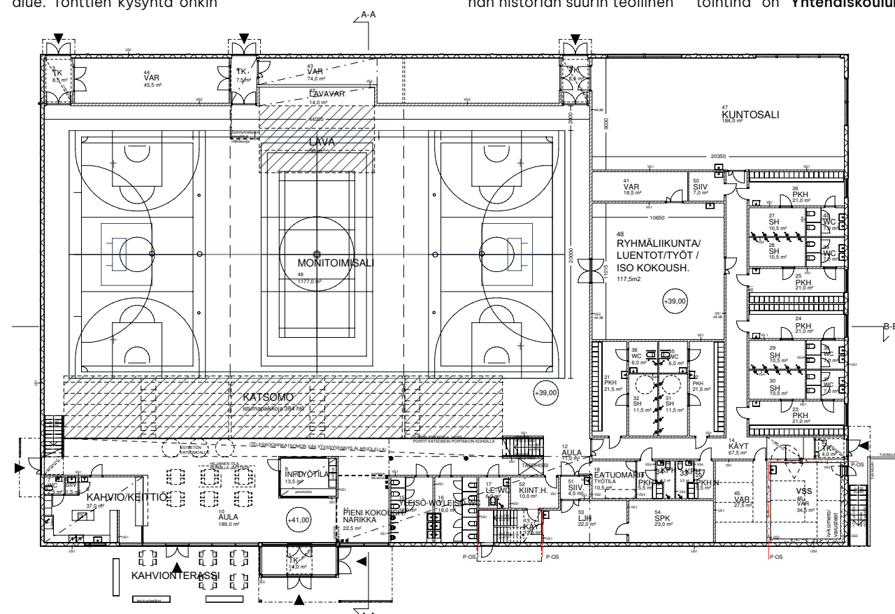
Monitoimihallin pohjakuva
