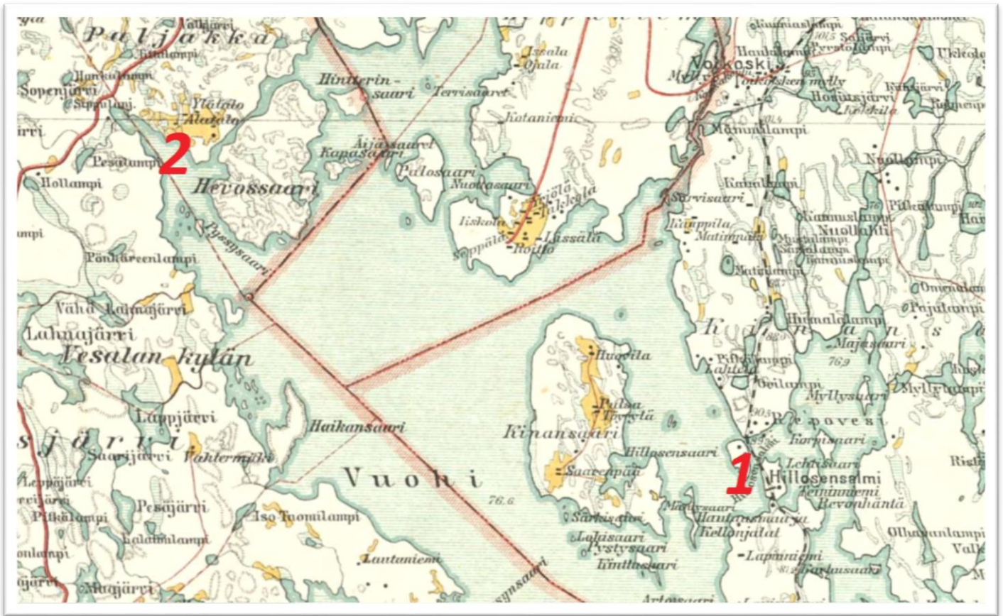
Karttaan merkittynä Hillosensalmen rautatieasema (1) ja Paljakanlahti (2) jossa Veli Tissari oli Savon jäkäreiden mukana kohtalokkaassa punaisten suorittamassa väijytyksessä. Pohja: Suomen taloudellinen kartta 1920.
