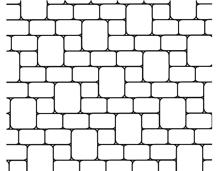
Klassikkokivet 60 mm, sekaladonta Kivien menekki: Klassikko neliötä 2/17, suorakaidetta 9/17 ja isoa suorakaidetta 6/17 pinta-alasta
