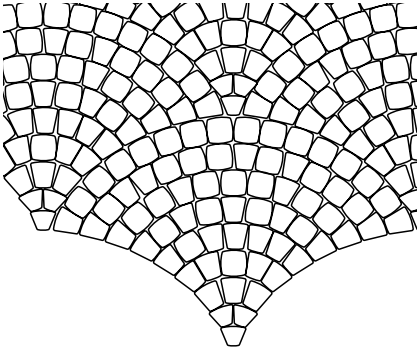
Klassikkokivet 60 mm, suomuladonta Yhteensä kuvioon menee 3 kpl pientä kaarretta, 30 kpl suurta kaarretta ja 35 kpl Klassikko neliötä. 1 suomu yht. 0,82 m 2
