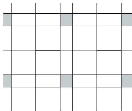
278 x 138 mm (8/25 pinta-alasta), 138 x 138 mm (1/25 pinta-alasta) ja 278 x 278 mm (16/25 pinta-alasta) + kahden reunan oikaisuun 138 x 138 mm ja 278 x 138 mm.
