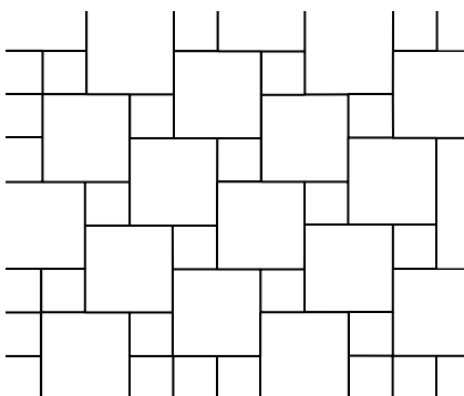
138 x 138 mm (1/5 pinta-alasta) ja 278 x 278 mm (4/5 pinta-alasta)
