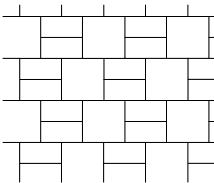
Kartanokivi ja Kartanolaatta Betonilaatat 418x208 ja 418x418 tai graniit- tilaatat 415x205 ja 415x415 mm
