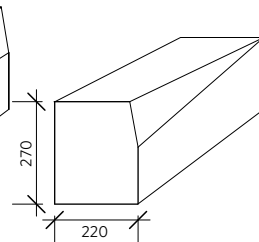
Sovitekivi, laskee oikealle
