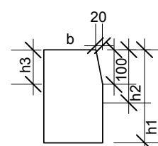
Viistereunakivi (V) sahattu
