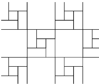
Kartanokivi, Linnakivi ja Betonilaatta 418 x 418 mm kivien menekki: Kartanokiviä 8/18, Linnakiviä 1/18 ja laattaa 1/2 pinta-alasta
