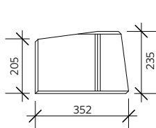
Peruskaarre ja kaarekans
