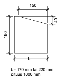
Luiskattu reunakivi (LR)
